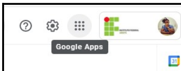
Imagem 1: “Google Apps”
