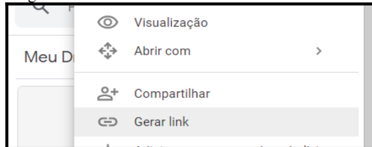
Imagem 3: Gerar link
