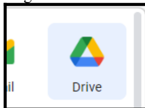
Imagem 2: Drive
