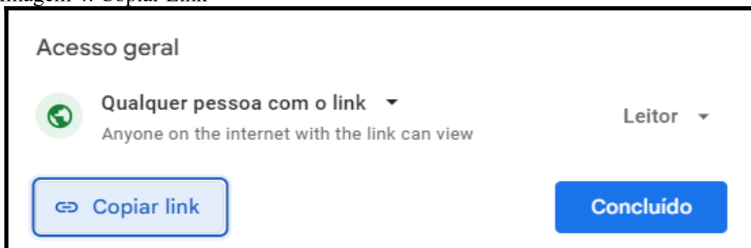
Imagem 4: Copiar Link
